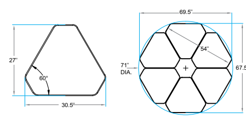
Model 03083. Interchange Mini Diamond Student Desk
