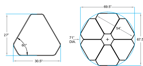
Model 04505. Interchange Mini Diamond Student Desk
